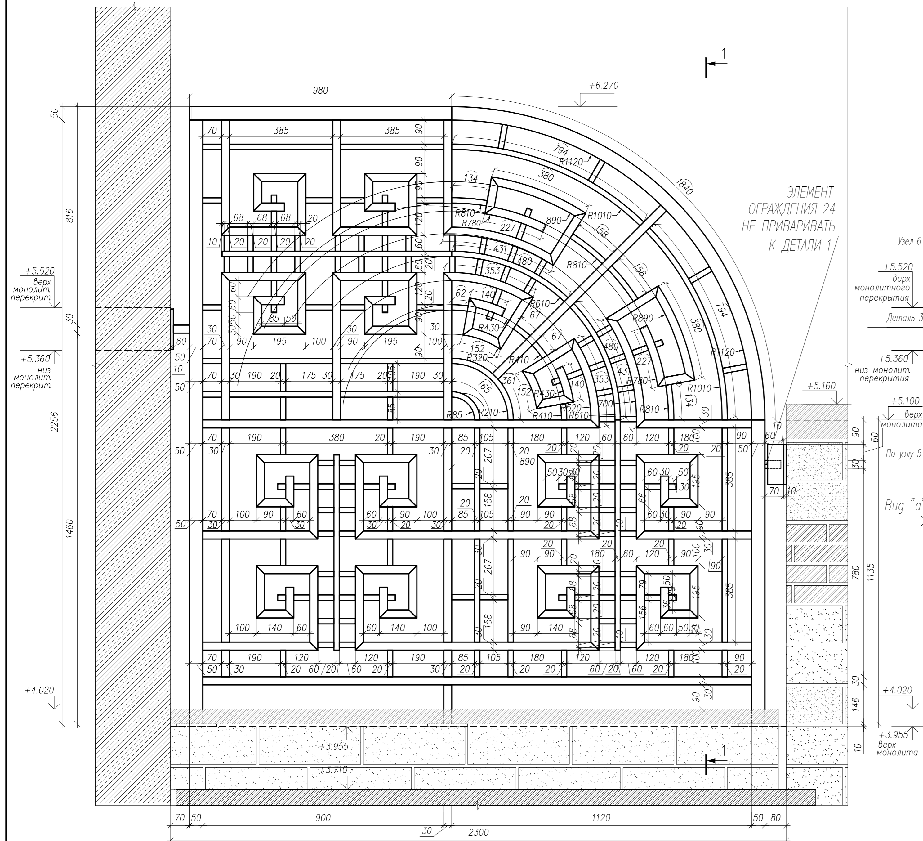
Металлическое ограждение ОГ-2. Вид А
