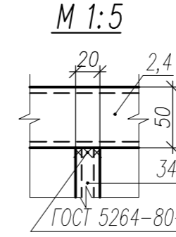
Узел 10 М 1:5
