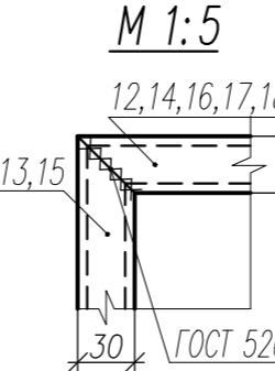
Узел 9 М 1:5
