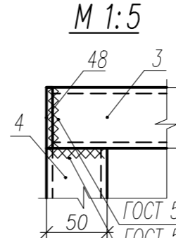
Узел 7 М 1:5
